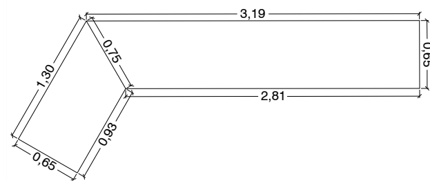
PLANTA BAIXA 1:50
