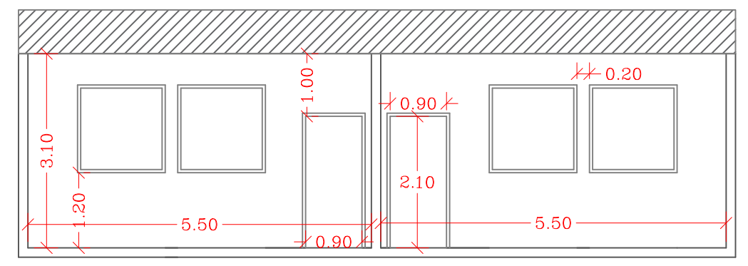
CORTE B-B 1:50
