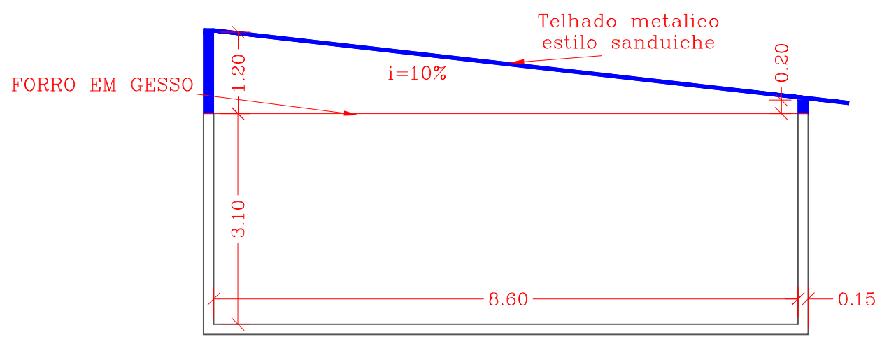
CORTE A-A 1:50
